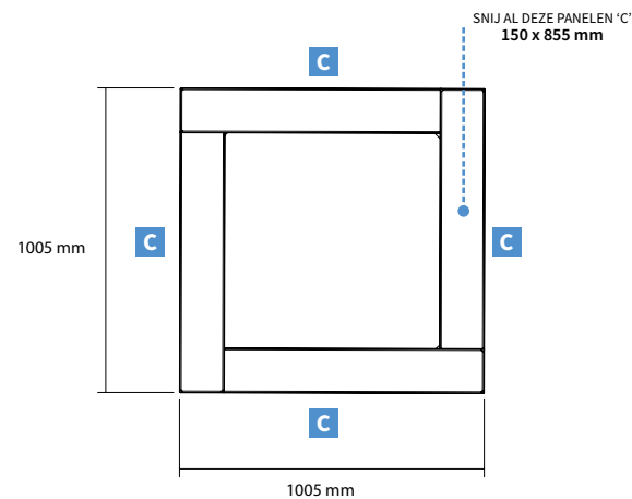
Bovenaanzicht
