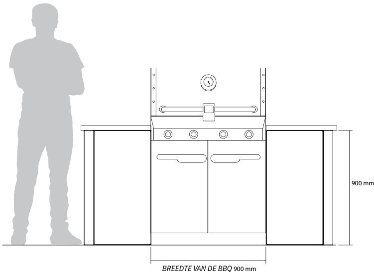
Voorraanzicht
