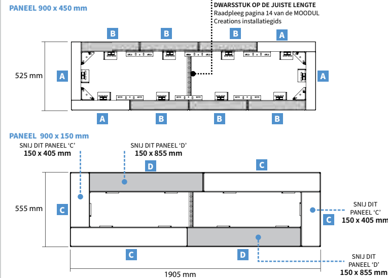
Bovenaanzicht
