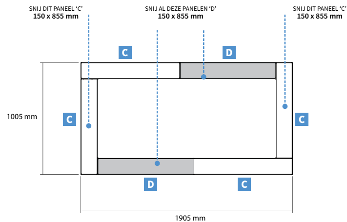
Bovenaanzicht
