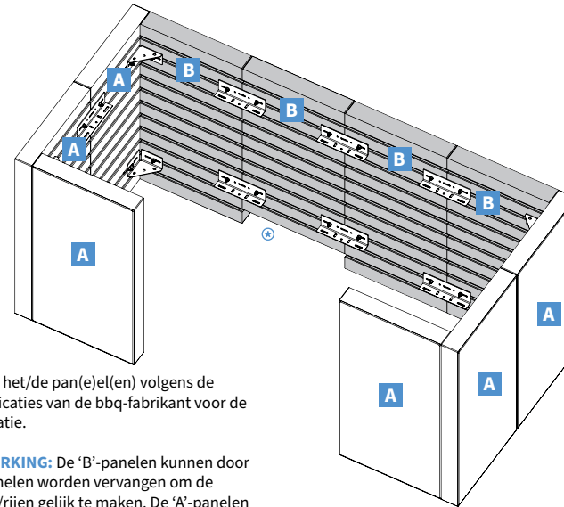
Binnenaanzicht
