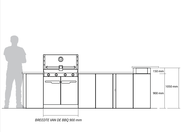
Vooraanzicht
