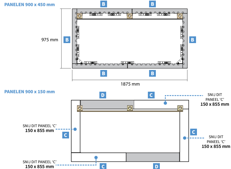
Bovenaanzicht
