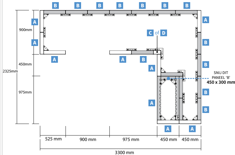
Bovenaanzicht
