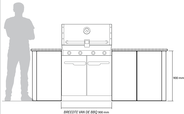
Voorraanzicht
