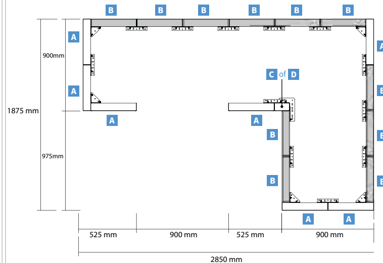
Bovenaanzicht
