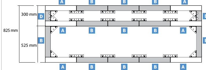
Bovenaanzicht
