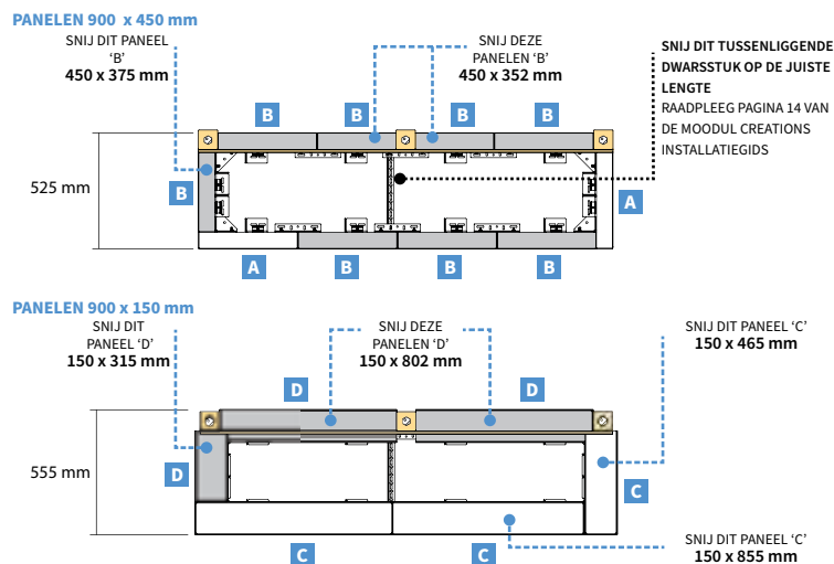
Bovenaanzicht
