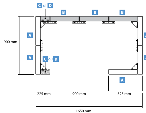
Bovenaanzicht
