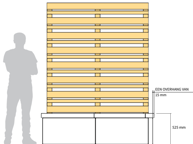
Vooraanzicht
