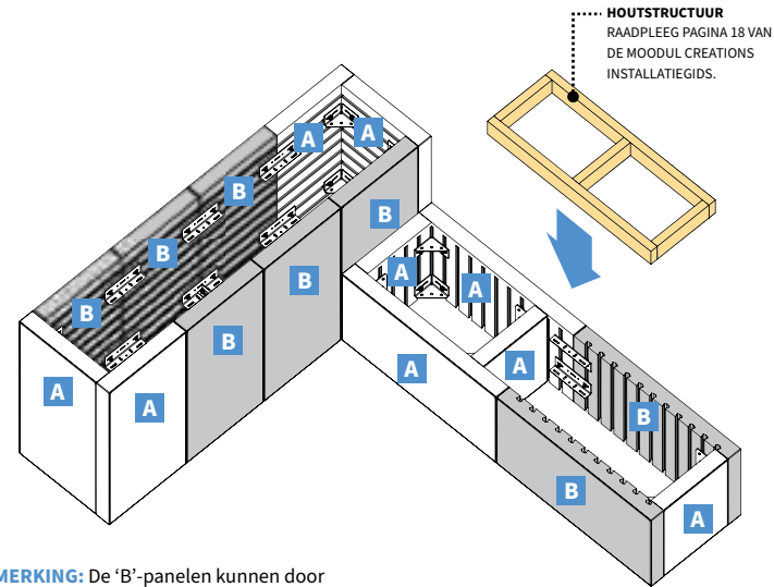
Binnenaanzicht
