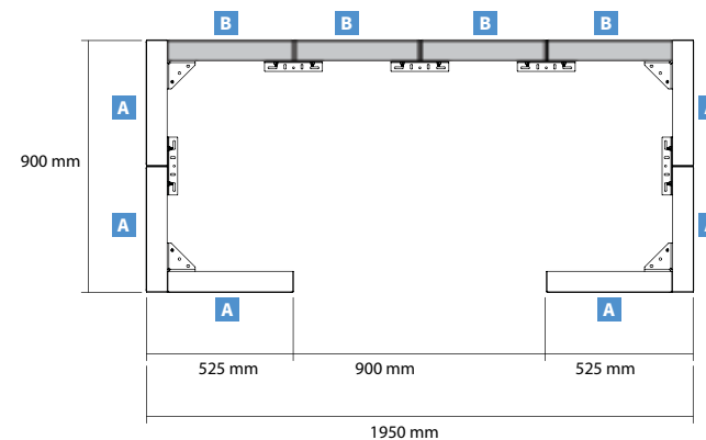
Bovenaanzicht
