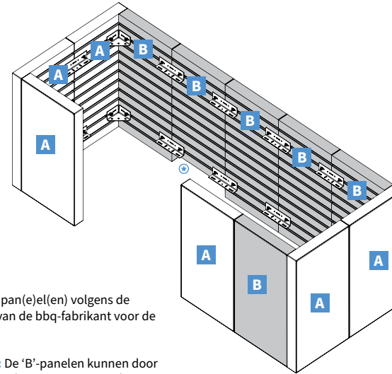
Binnenaanzicht
