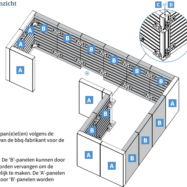
Binnenaanzicht
