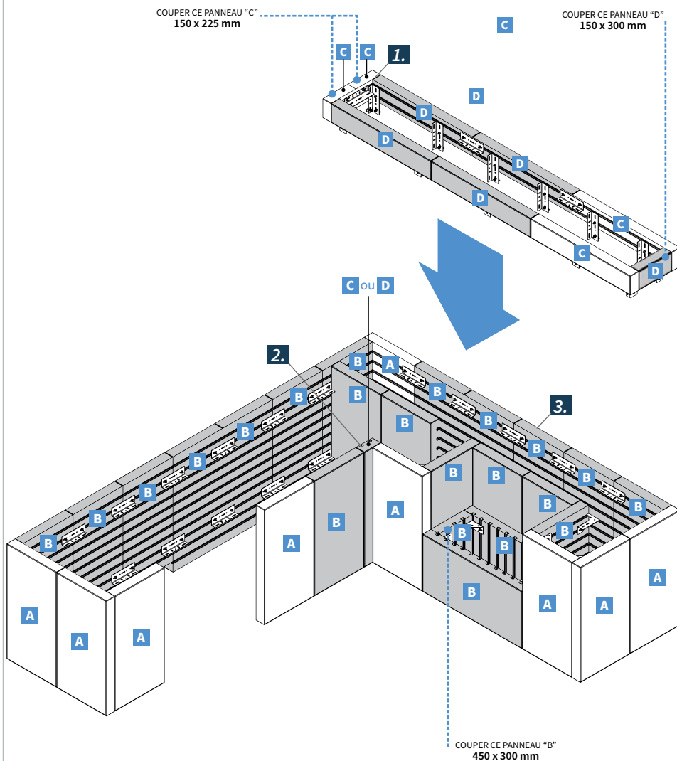
Vue éclatée
