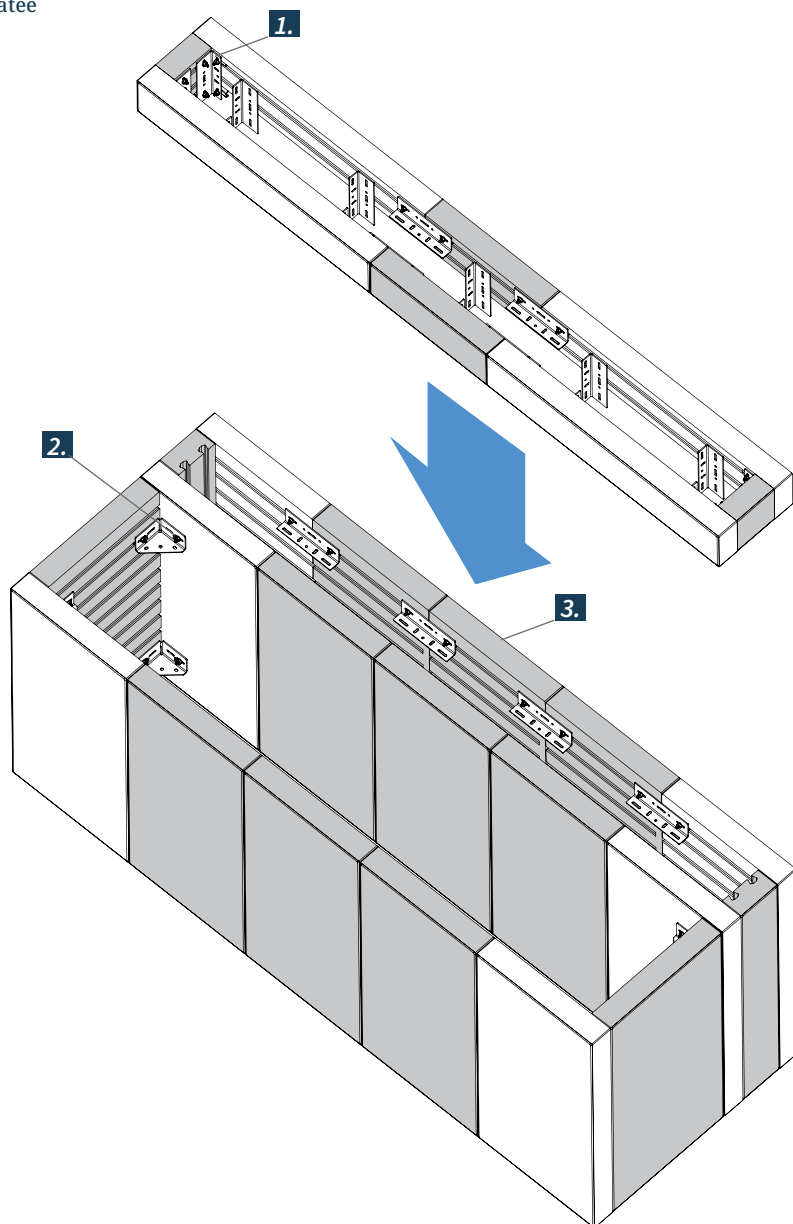
Vue éclatée
