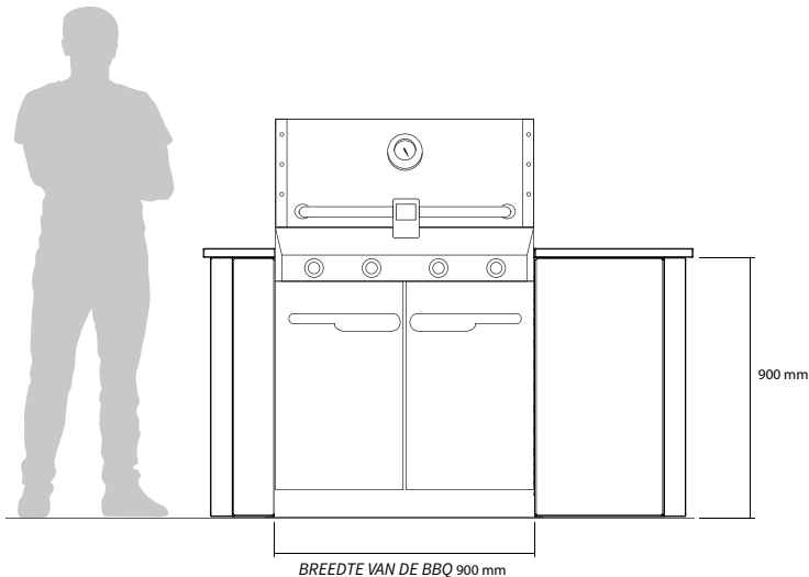
Vooraanzicht
