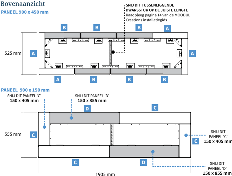
Bovenaanzicht
