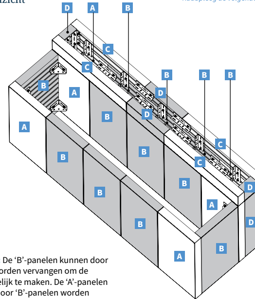
Binnenaanzicht
