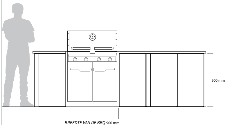
Vooraanzicht
