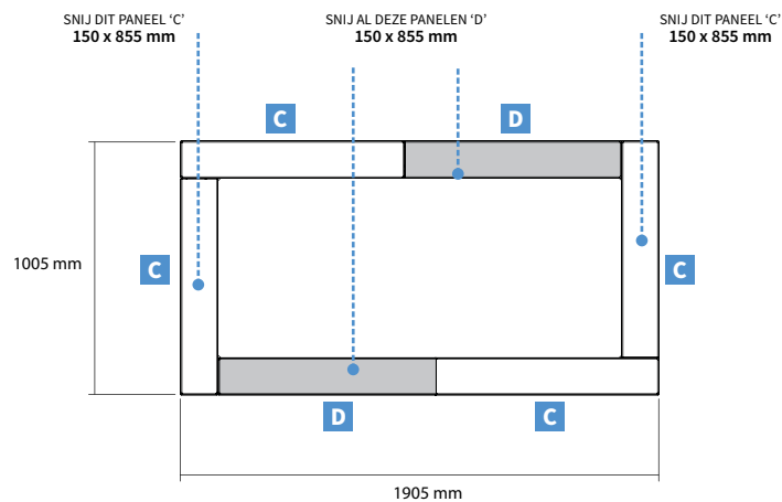
Bovenaanzicht
