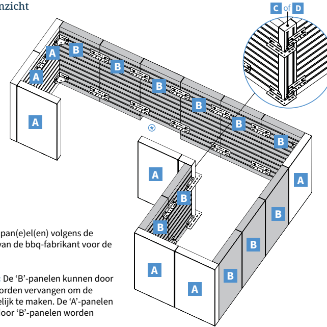
Binnenaanzicht
