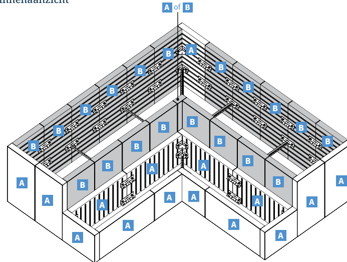
Binnenaanzicht
