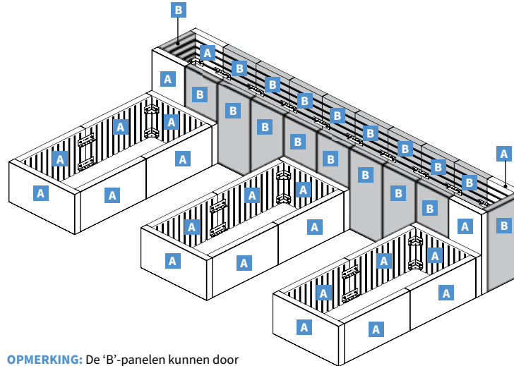
Binnenaanzicht
