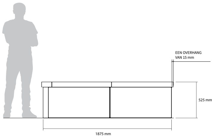
Vooraanzicht
