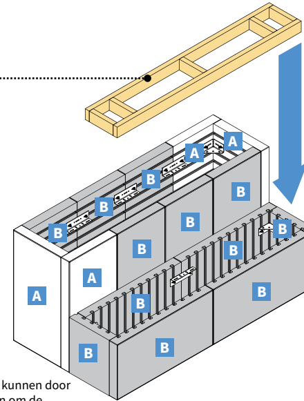
Binnenaanzicht
