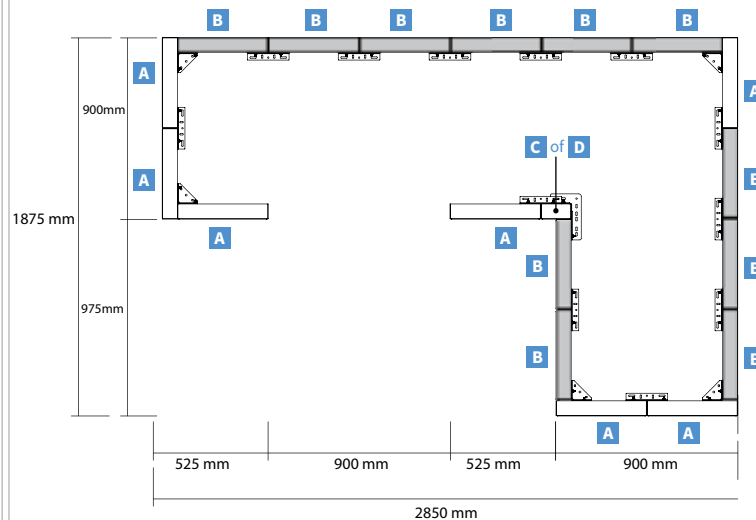
Bovenaanzicht
