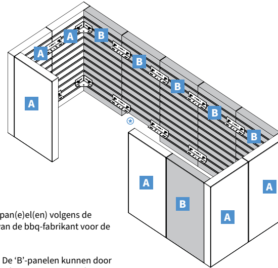
Binnenaanzicht
