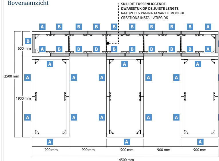
Bovenaanzicht
