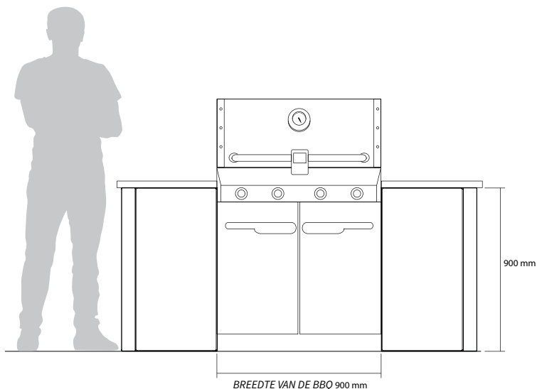
Vooraanzicht
