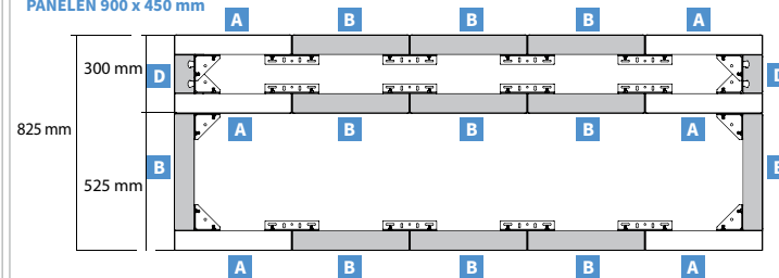
Bovenaanzicht
