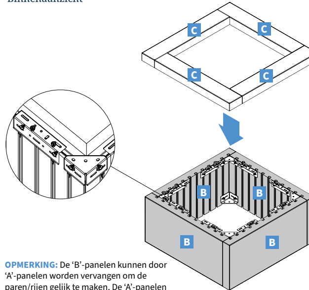
Binnenaanzicht
