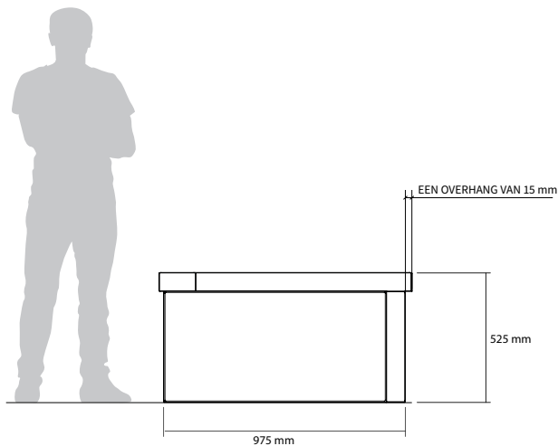
Vooraanzicht
