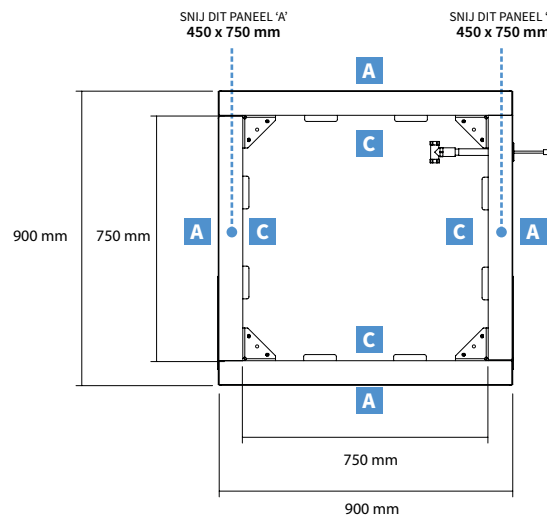
Bovenaanzicht
