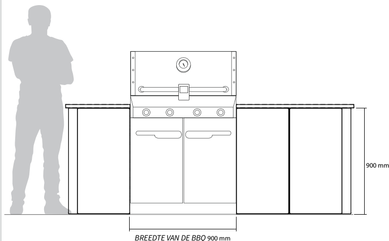
Vooraanzicht
