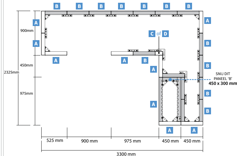
Bovenaanzicht
