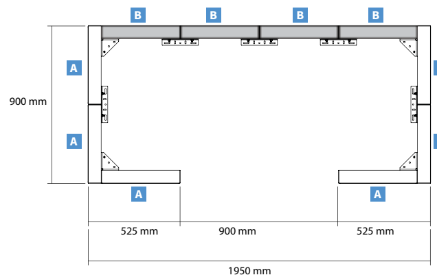
Bovenaanzicht
