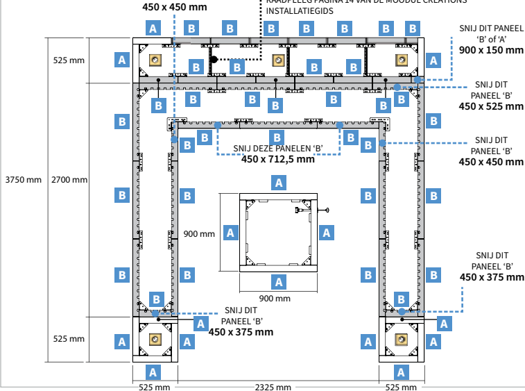
Bovenaanzicht
