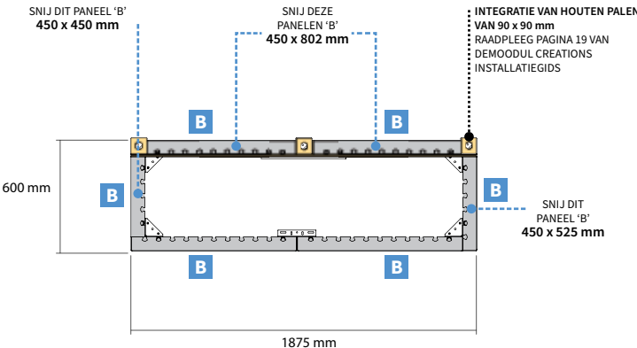
Bovenaanzicht
