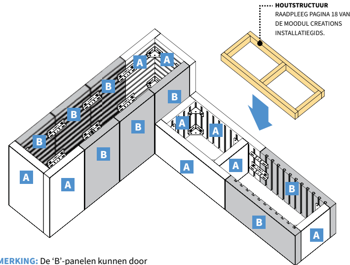
Binnenaanzicht
