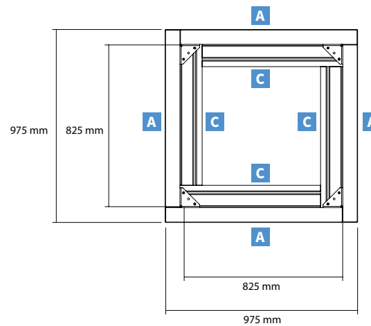
Bovenaanzicht
