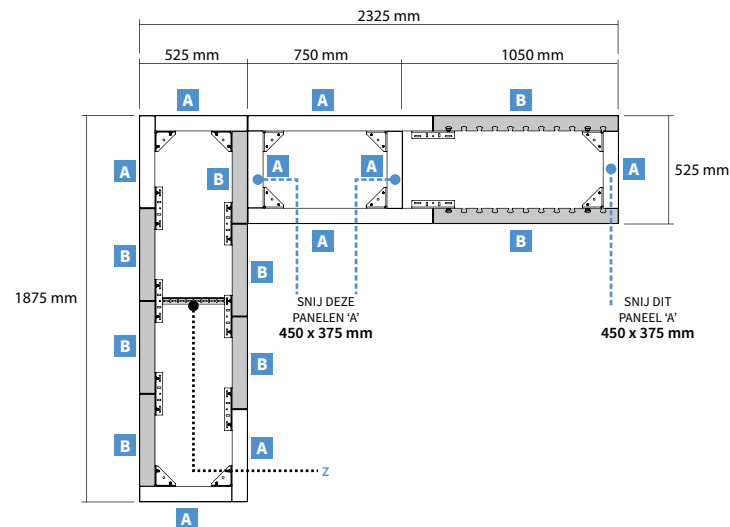
Bovenaanzicht
