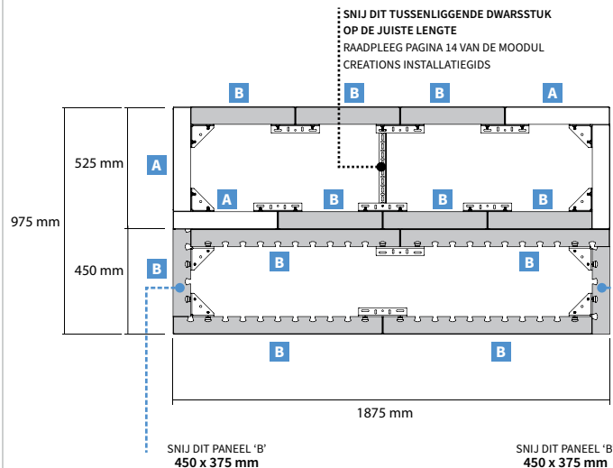
Bovenaanzicht
