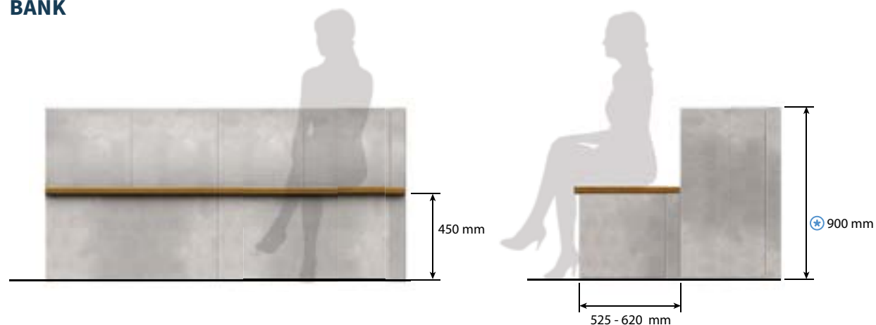
VOORAANZICHT
