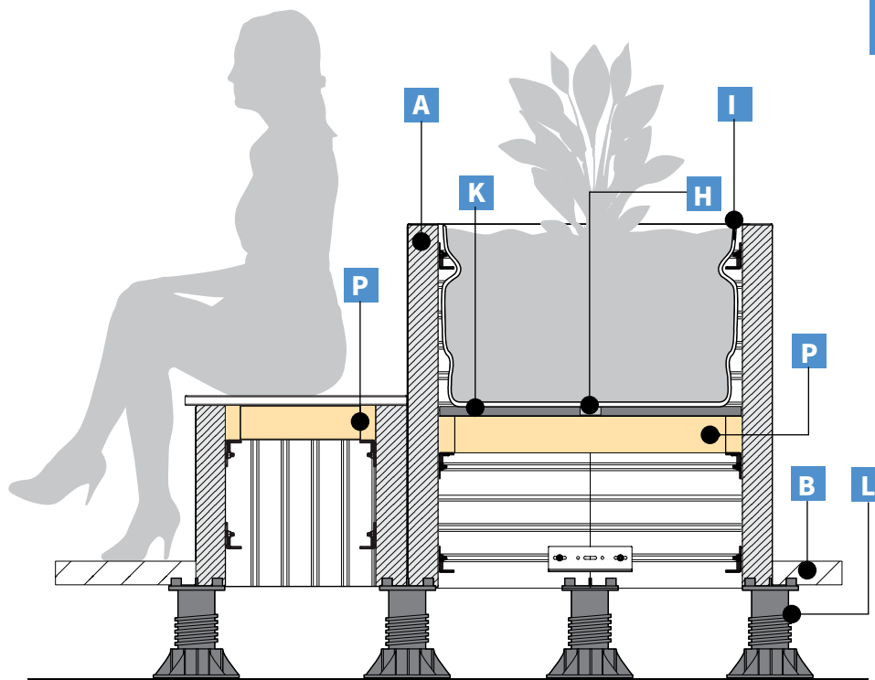
Bloembak geplaatst op tegeldragers - doorsnede
