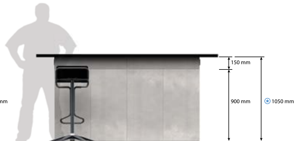
VOORAANZICHT
