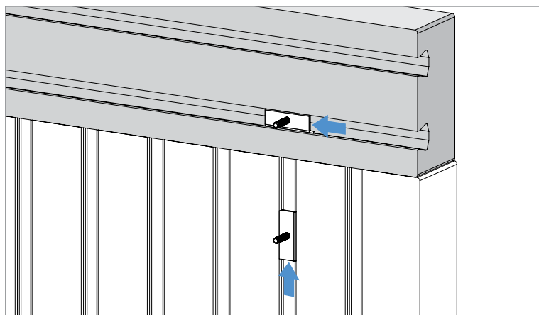
PANEEL 900 x 450 x 75 mm HORIZONTAAL GEMONTEERD
