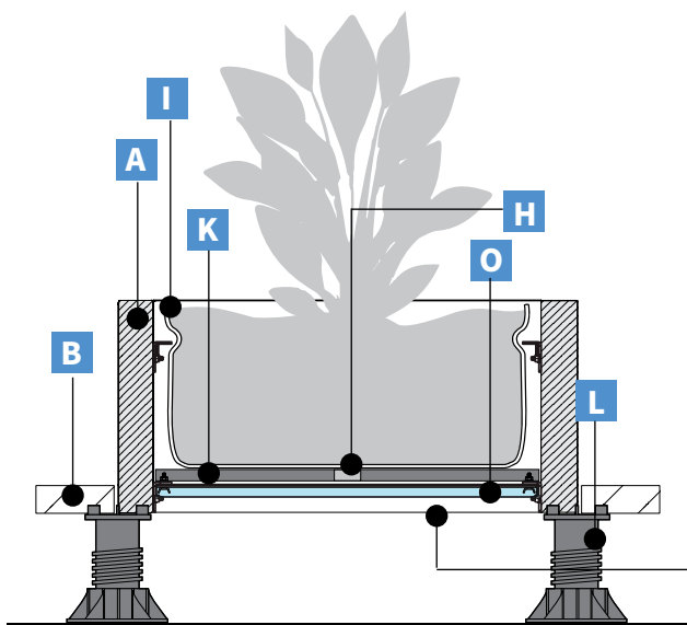
Bloembak geplaatst op tegeldragers - doorsnede
